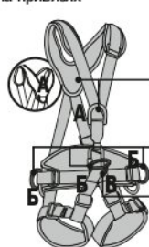
Рис. 3. Расположение и назначение крепежных точек на привязях
