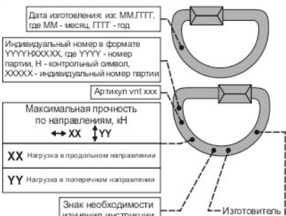
Рис. 2. Идентификация и маркировка изделия
