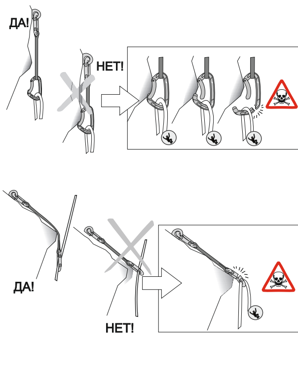
Рис. 4. Установка оттяжек
