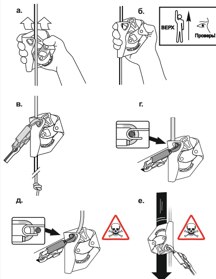
Рис. 4. Установка зажима на канат
