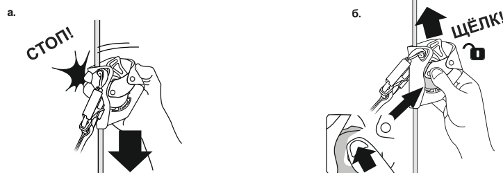
Рис. 6. Функциональная проверка зажима
