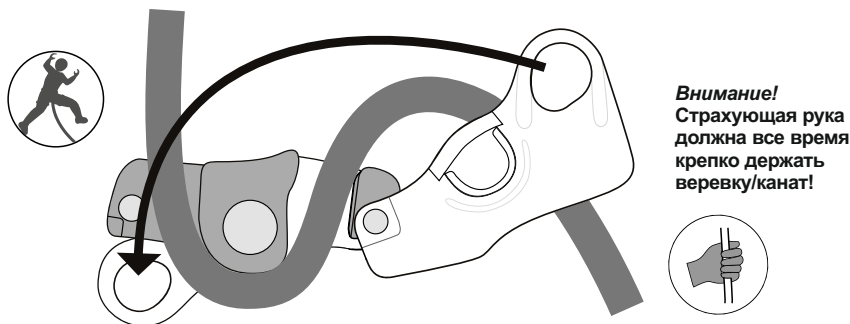
Рис. 5. Заправка веревки в страховочное устройство
