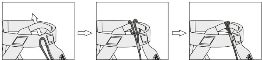
Рис. 5. Крепление усов самостраховки
