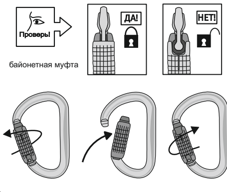
Рис. 3. Открытие / закрытие / фиксация карабина
