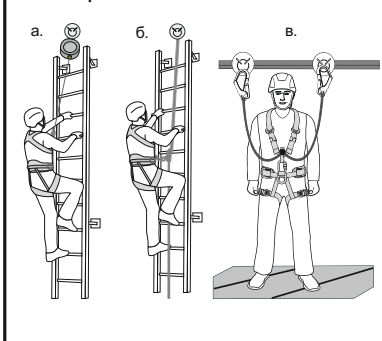
Рис. 8. Страховочная система
