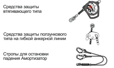
Рис. 9. Соединительно-амортизирующая подсистема
