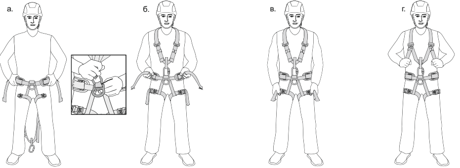
Рис. 5. Надевание привязи
