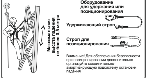
Рис. 10. Позиционирование в рабочем положении
