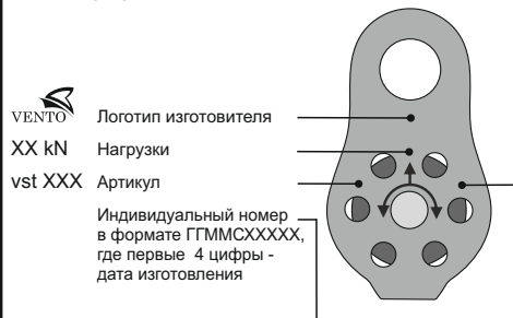
Рис. 2. Маркировка изделий
