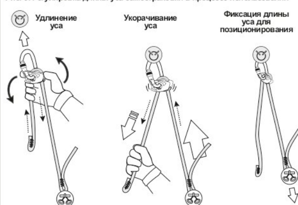
Рис. 9. Регулировка длины уса самостраховки в процессе использования
