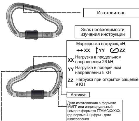
Рис. 2. Маркировка изделий
