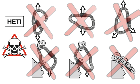
Рис. 5. Недопустимое использование
