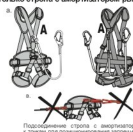
Рис. 5. В страховочных системах допускается использование только стропа с амортизатором рывка
