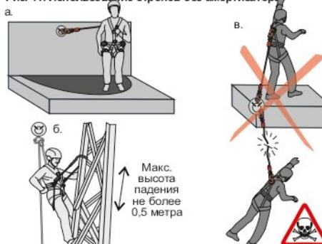
Рис. 11. Использование стропов без амортизатора
